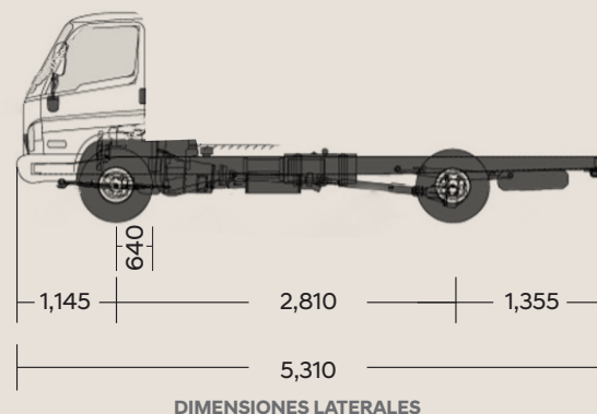
DIMENSIONES LATERALES
