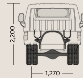
DIMENSIONES FRONTAL Y POSTERIOR
