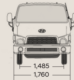
DIMENSIONES FRONTAL Y POSTERIOR
